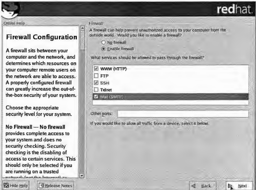
Imagen 14: Configuración del Firewall
