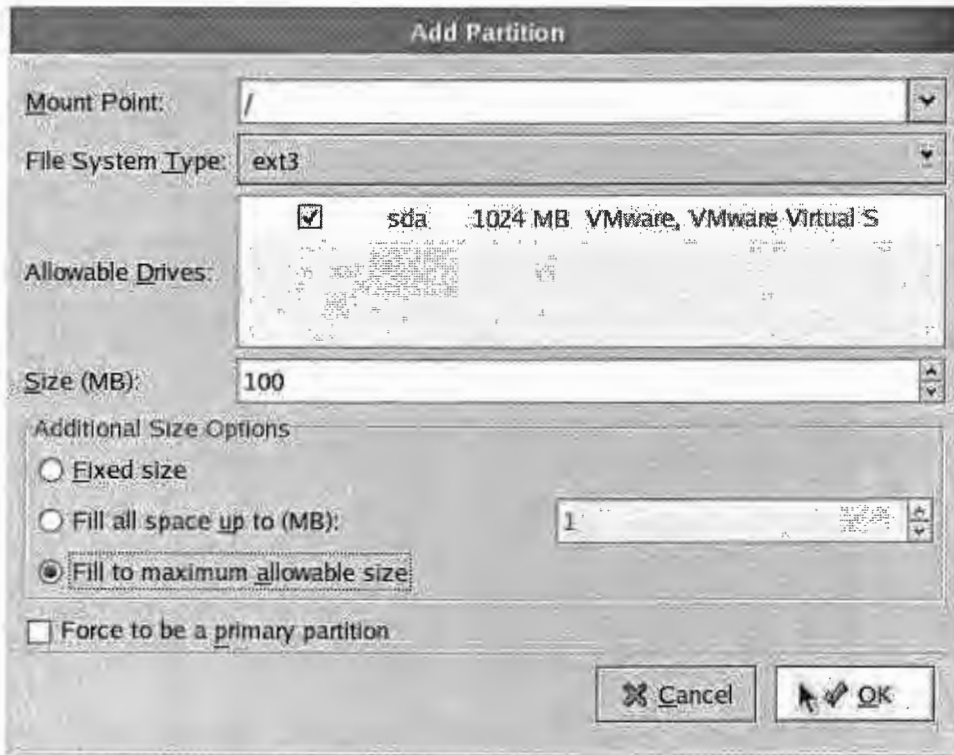
Imagen 11: Añadir Partición ext3
