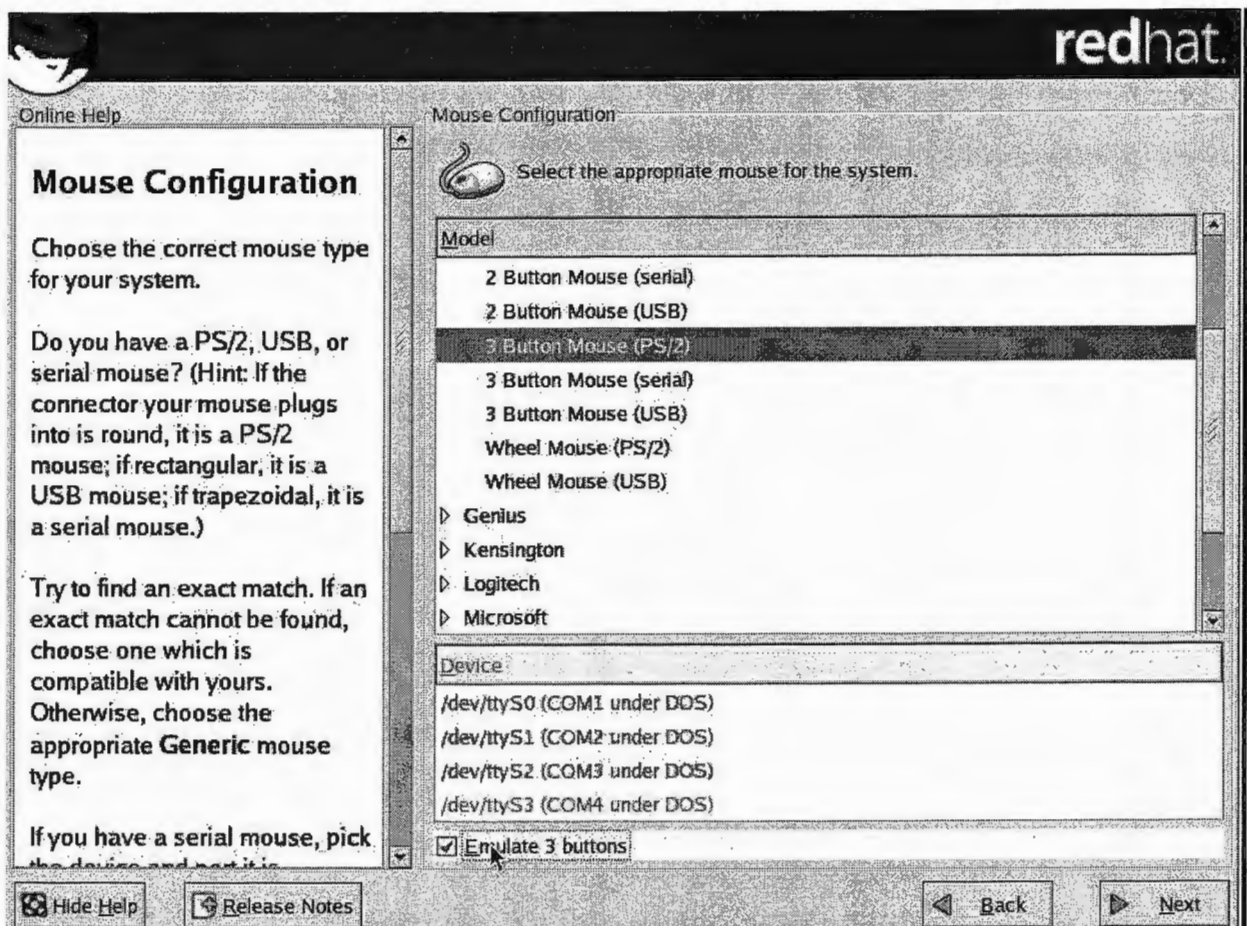
Imagen 5: Configuración del Mouse
