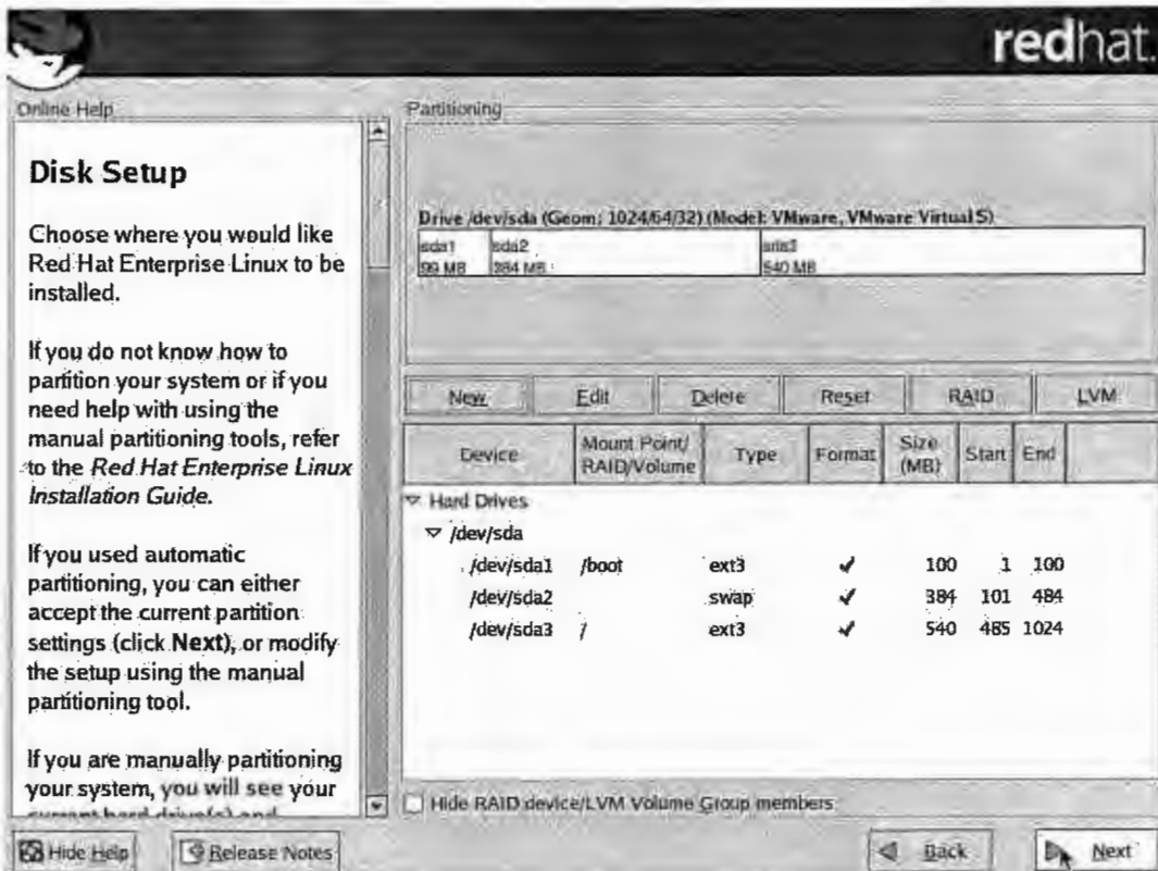
Imagen 12: Confirmación de Particiones Creadas
