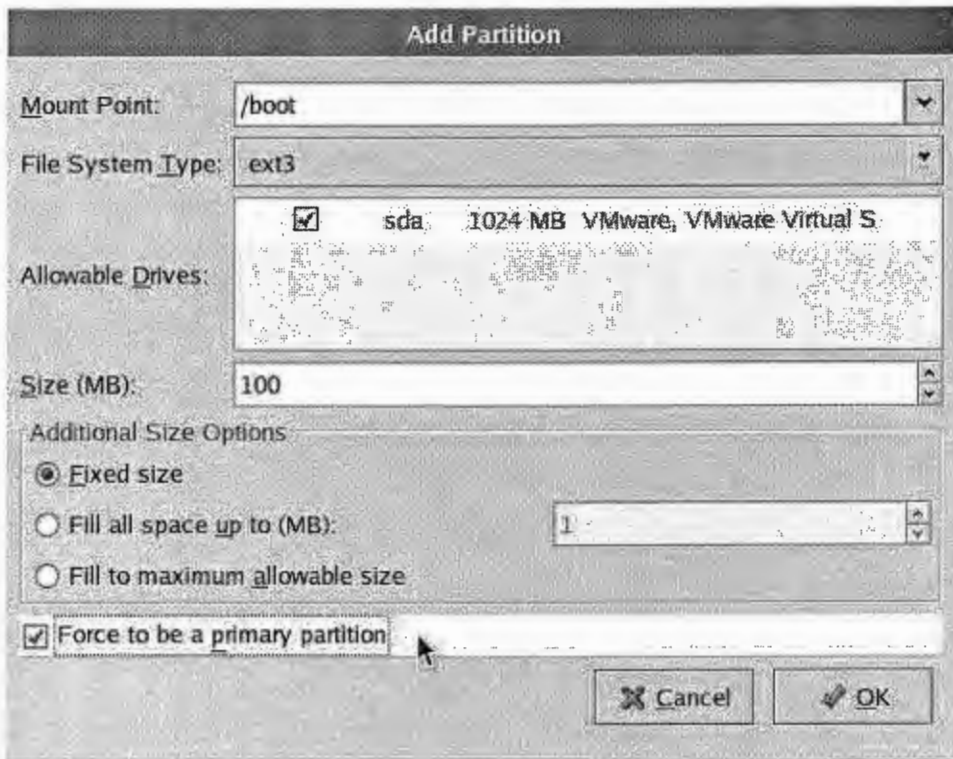
Imagen 9: Añadir Partición /boot
